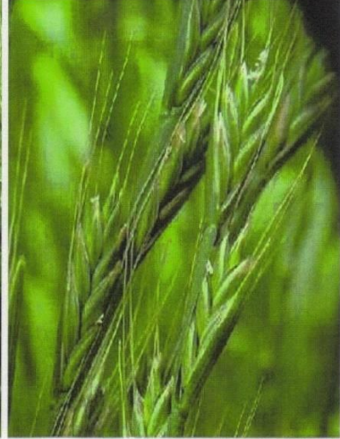
TARES: Lolium Temulentum
